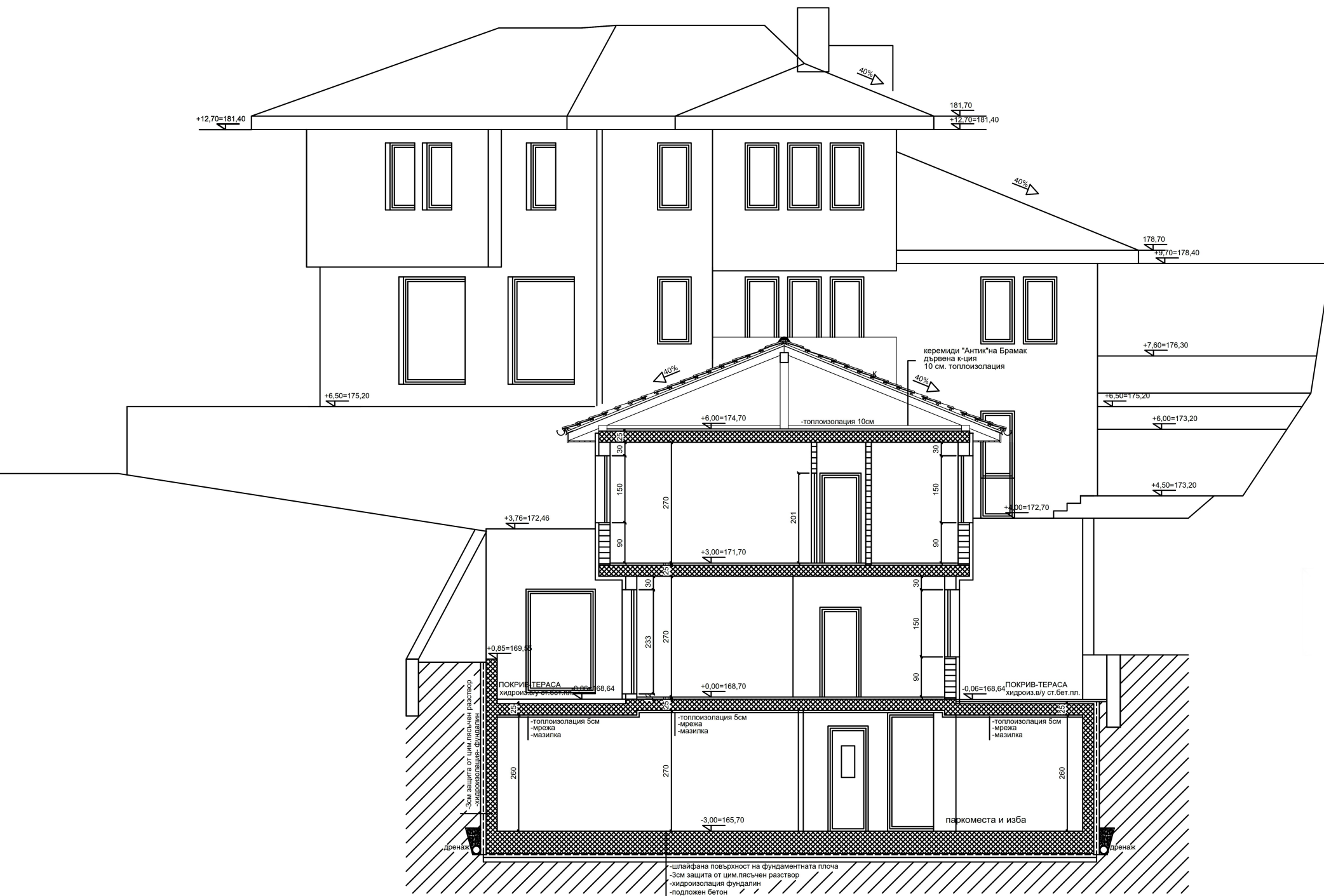
ВЕРТИКАЛЕН РАЗРЕЗ "С-С"
