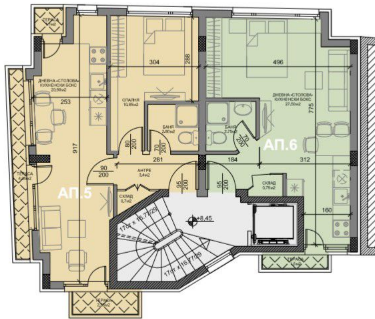
РАЗПРЕДЕЛЕНИЕ НА 4 ЕТАЖ
