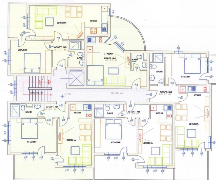
РАЗПРЕДЕЛЕНИЕ И ТЕХНОЛОГИЧНО ОБЗАВЕЖДАНЕ НА ВТОРИ ЖИЛИЩЕН ЕТАЖ М 1:50
