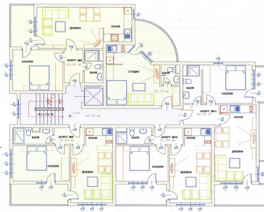
РАЗПРЕДЕЛЕНИЕ И ТЕХНОЛОГИЧНО ОБЗАВЕЖДАНЕ НА ТРЕТИ ЖИЛИЩЕН ЕТАЖ М 1:50
