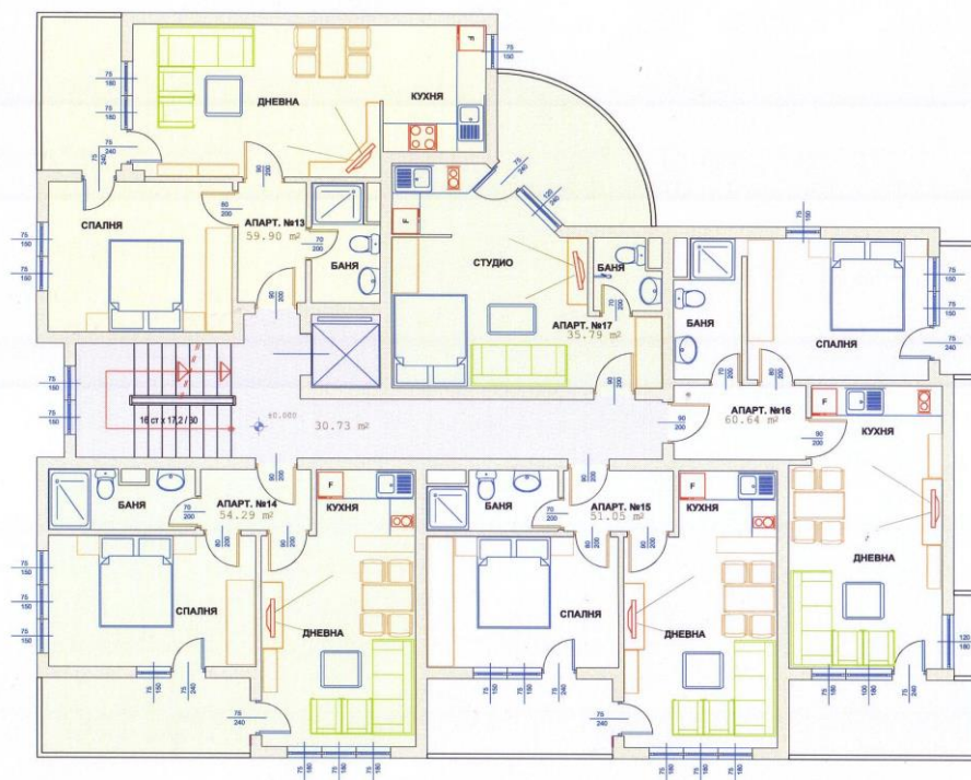
РАЗПРЕДЕЛЕНИЕ И ТЕХНОЛОГИЧНО ОБЗАВЕЖДАНЕ НА ЧЕТВЪРТИ ЖИЛИЩЕН ЕТАЖ М 1:50
