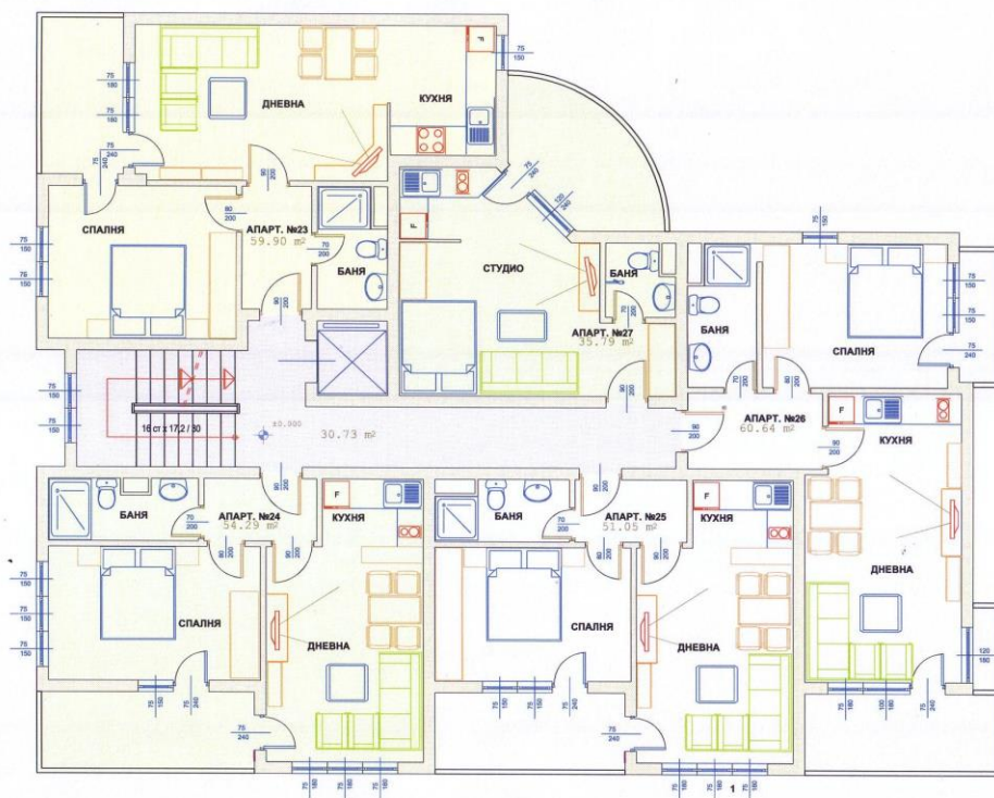
РАЗПРЕДЕЛЕНИЕ И ТЕХНОЛОГИЧНО ОБЗАВЕЖДАНЕ НА ШЕСТИ МАНСАРДЕН ЖИЛИЩЕН ЕТАЖ М 1:50
