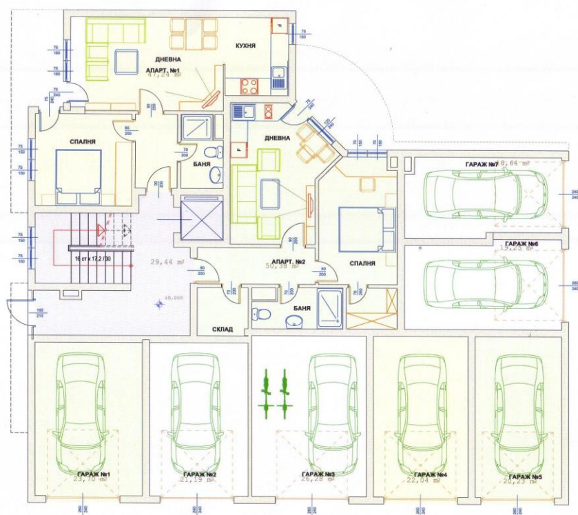
РАЗПРЕДЕЛЕНИЕ И ТЕХНОЛОГИЧНО ОБЗАВЕЖДАНЕ НА ПЪРВИ ПРИЗЕМЕН ЕТАЖ М 1:50
