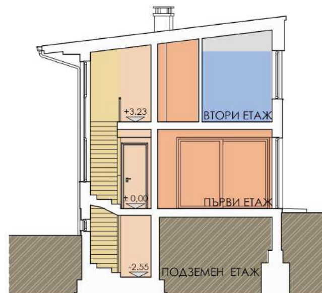
ВЕРТИКАЛЕН РАЗРЕЗ 2-2
