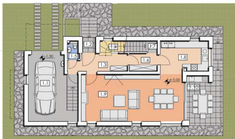
РАЗПРЕДЕЛЕНИЕ ПЪРВИ ЕТАЖ КОТИ -1,30 И ±0,00
