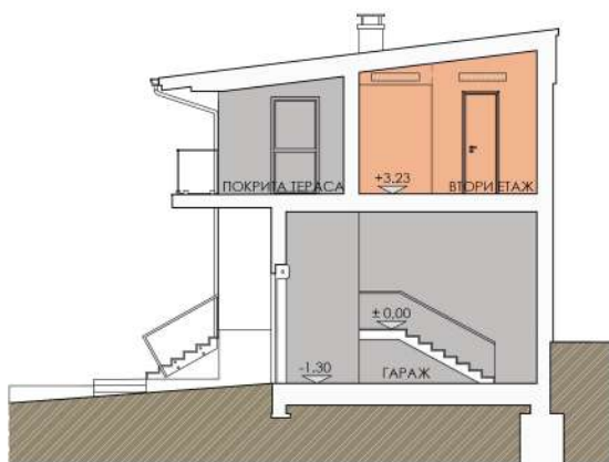
ВЕРТИКАЛЕН РАЗРЕЗ 1-1
