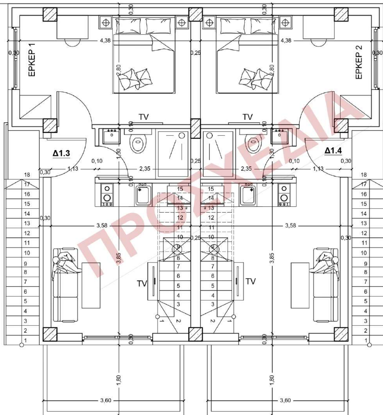
Κάτοψη ορόφου με ΕΡΚΕΡ
