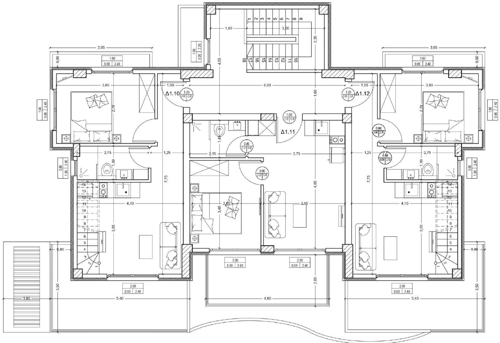
ΚΑΤΟΨΗ ΟΡΟΦΟΥ ΚΤΙΡΙΟΥ 2
