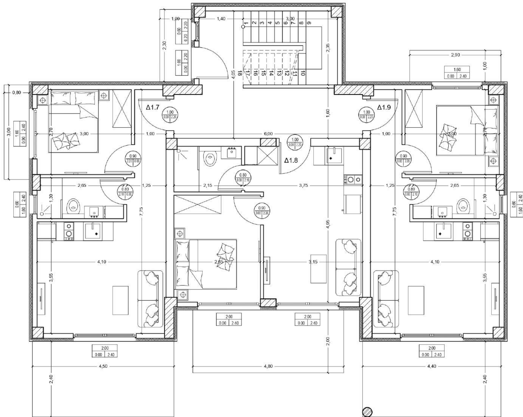
ΚΑΤΟΨΗ ΙΣΟΓΕΙΟΥ ΚΤΙΡΙΟΥ 2
