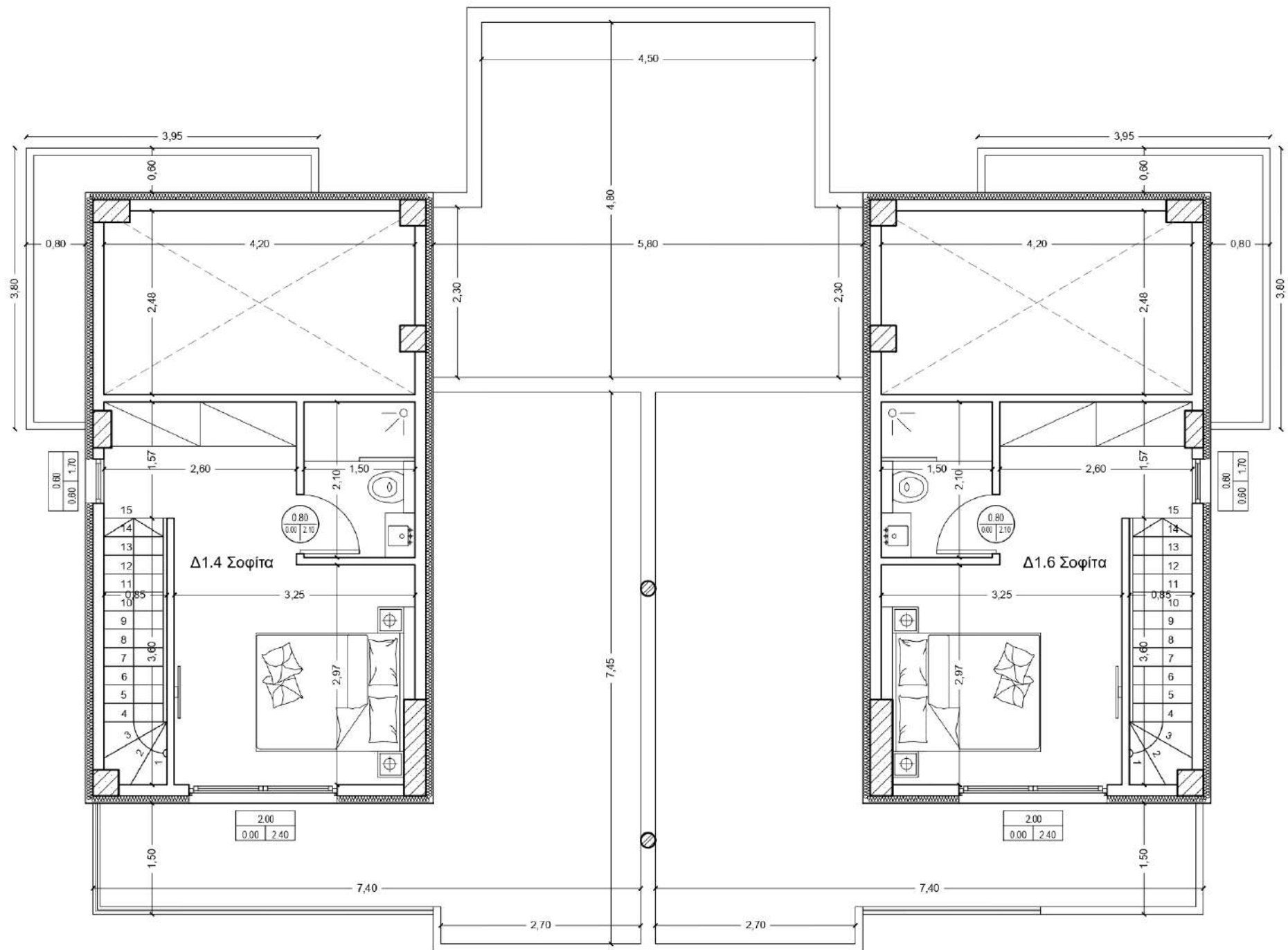
ΚΑΤΟΨΗ ΣΟΦΙΤΩΝ ΚΤΙΡΙΟΥ 1
