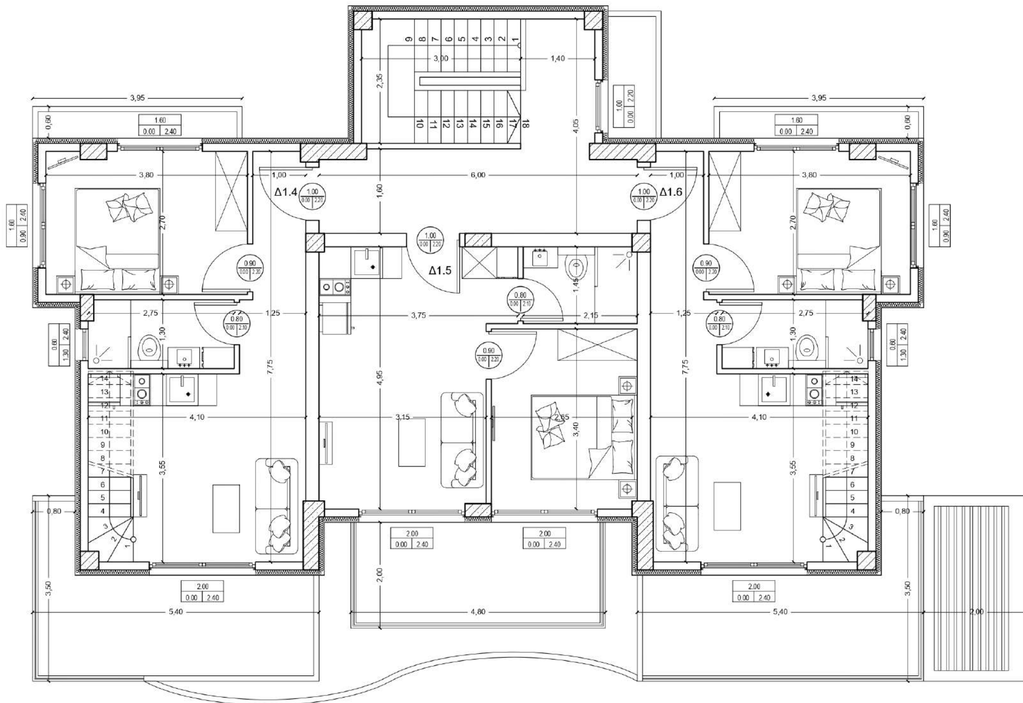
ΚΑΤΟΨΗ ΟΡΟΦΟΥ ΚΤΙΡΙΟΥ 1
