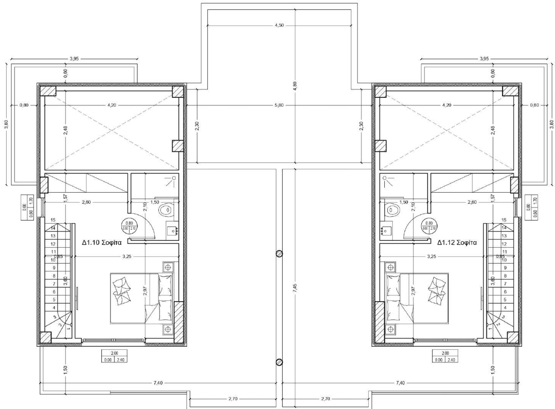
ΚΑΤΟΨΗ ΣΟΦΙΤΩΝ ΚΤΙΡΙΟΥ 2
