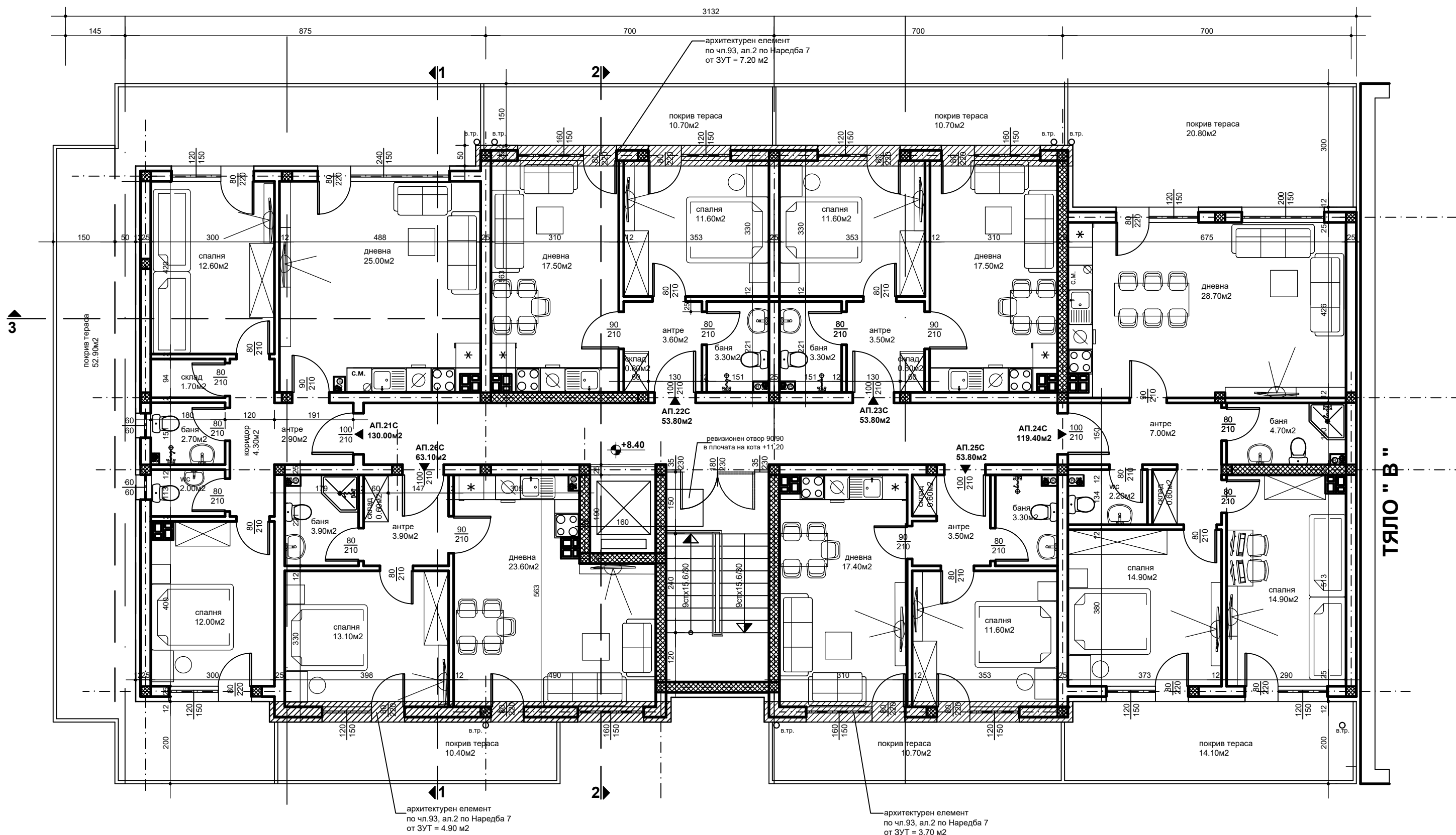
РАЗПРЕДЕЛЕНИЕ мансарден етаж ТЯЛО " С " 3.П. 524.00м2 М 1:50
