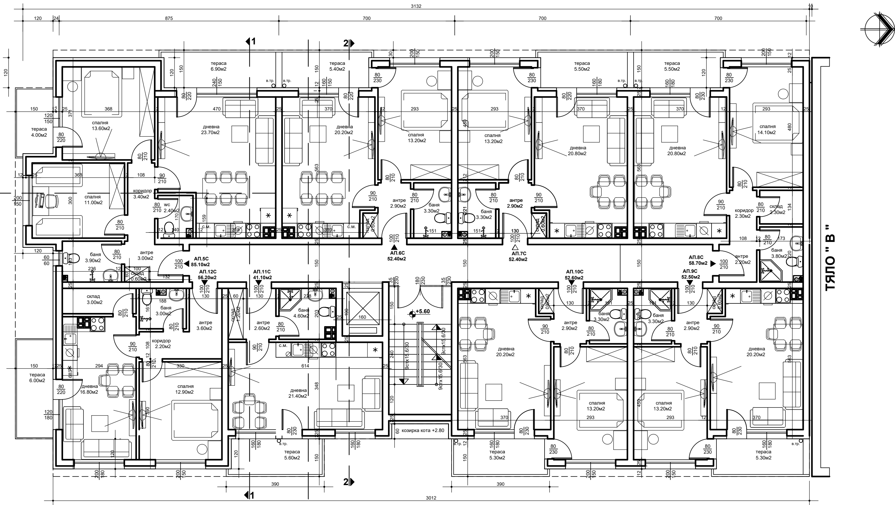
РАЗПРЕДЕЛЕНИЕ 2 ТЯЛО "С" 3.П. 510.70м2 М 1:50
