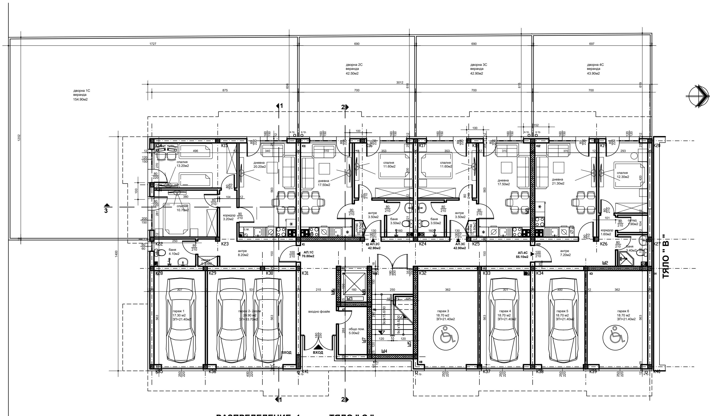
РАЗПРЕДЕЛЕНИЕ 1 этаж ТЯЛО " С " З.П. 421.70м 2 М 1:50 Р.З.П. ТЯЛО С - 1970.60м 2
