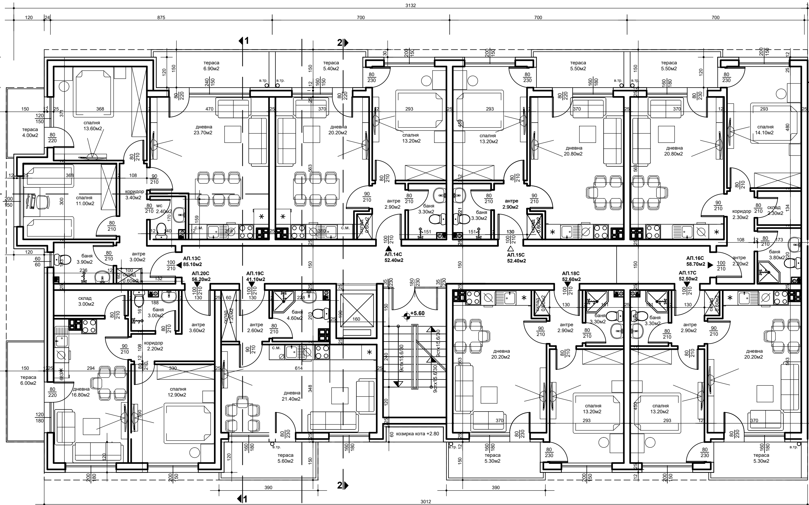
РАЗПРЕДЕЛЕНИЕ 3 етаж ТЯЛО " С " 3.П. 509.30м2 М 1:50
