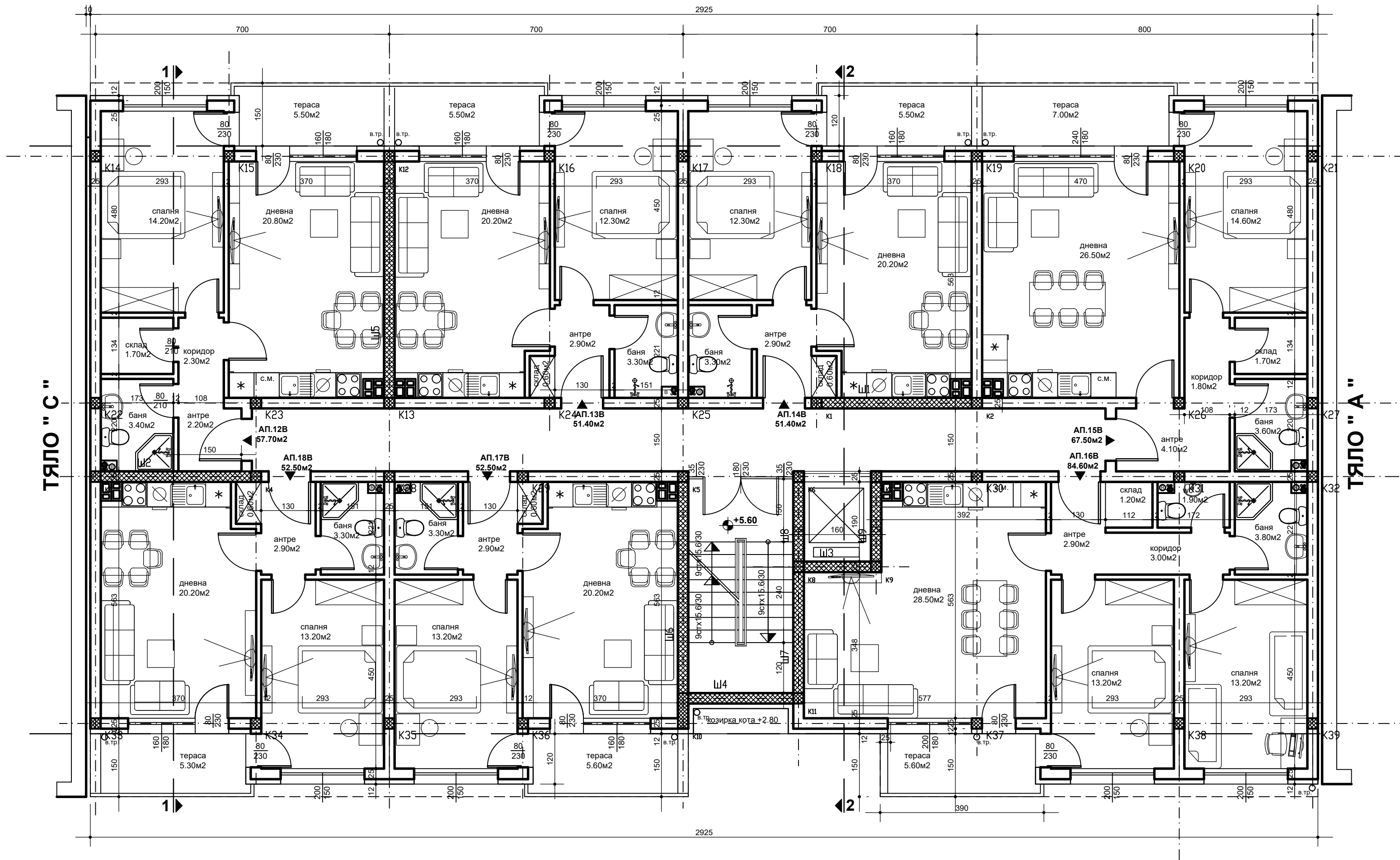
РАЗПРЕДЕЛЕНИЕ 3 этаж ТЯЛО " В " З.П. 481.20м² М 1:50
