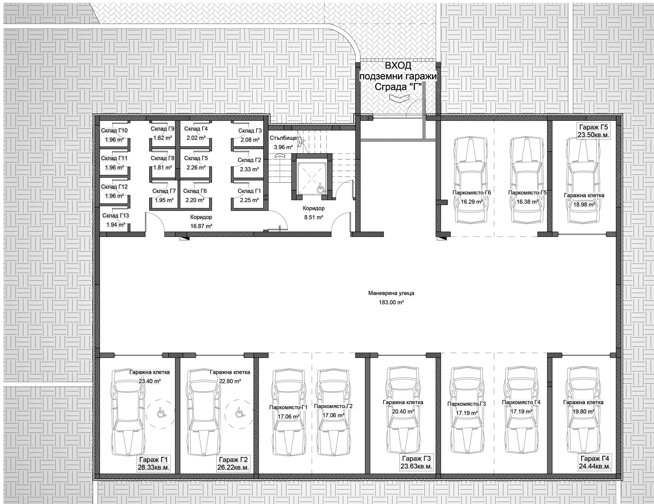
СГРАДА Г - РАЗПРЕДЕЛЕНИЕ НА СУТЕРЕН М 1:100
