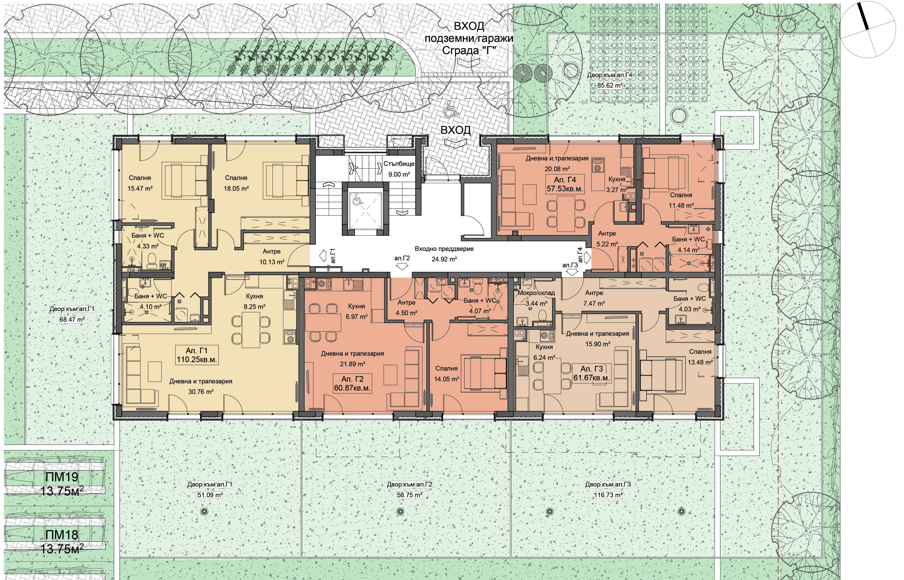
СГРАДА Г - РАЗПРЕДЕЛЕНИЕ НА ПЪРВИ ЕТАЖ М 1:100
