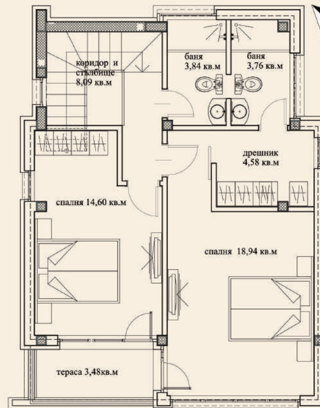
РАЗПРЕДЕЛЕНИЕ II-ри етаж, кота +3,15 ЗП 73,61 кв. м.
