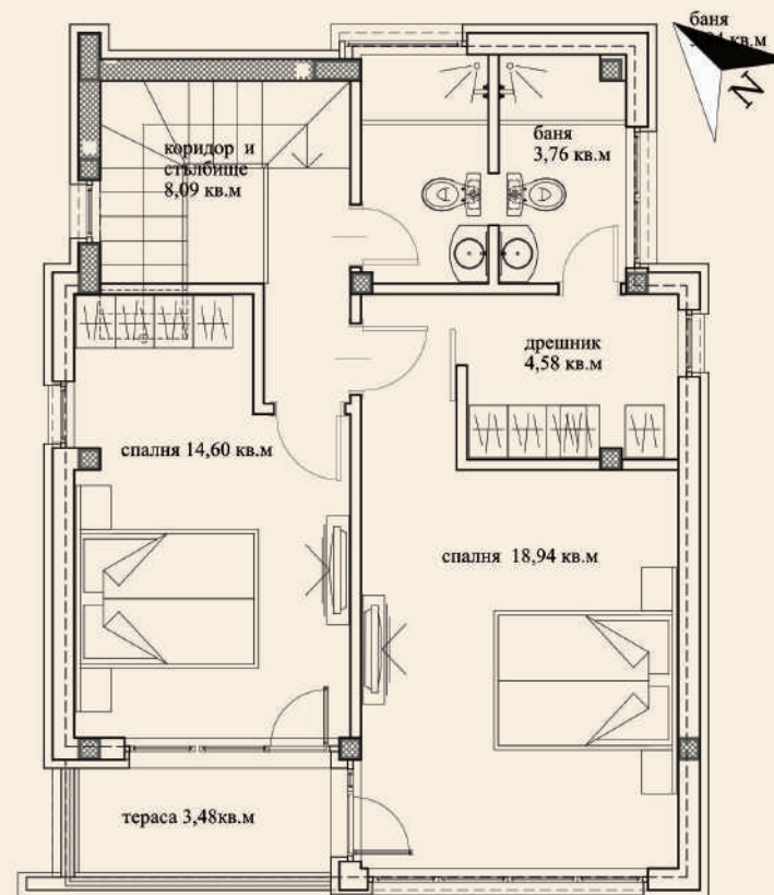
РАЗПРЕДЕЛЕНИЕ II-ри етаж, кота +3,15 ЗП 73,61 кв. м.
