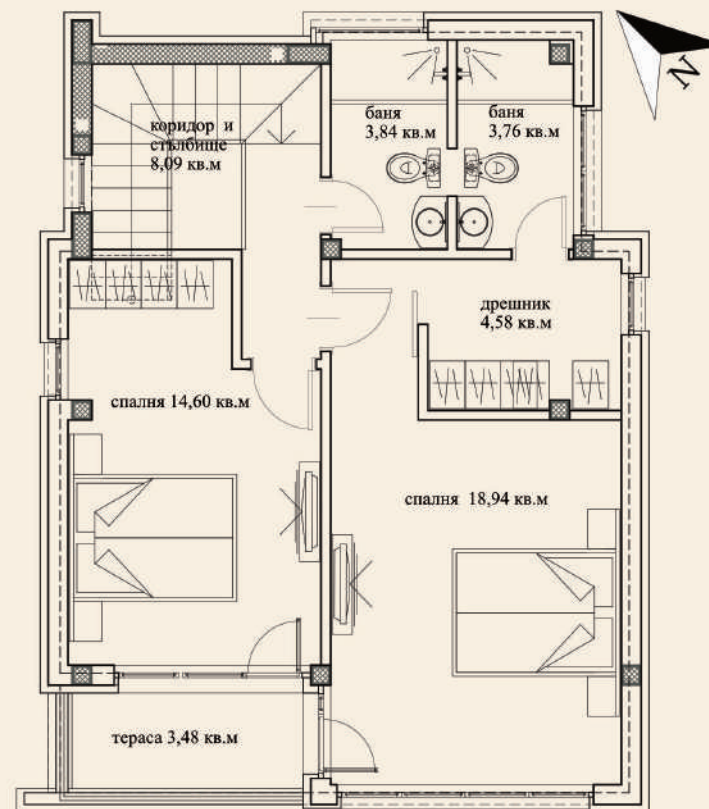
РАЗПРЕДЕЛЕНИЕ II-ри етаж, кота +3,15 ЗП 73,61 кв. м.
