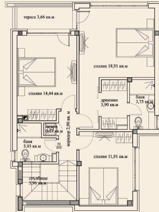
РАЗПРЕДЕЛЕНИЕ II-ри етаж, кота +3.15 ЗП 88,70 кв. м.
