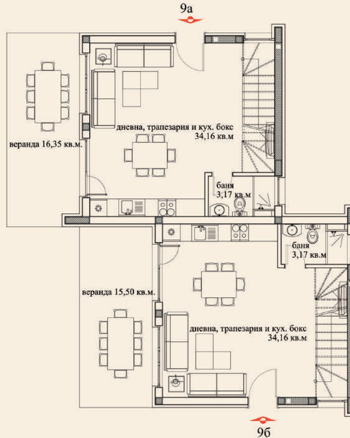
РАЗПРЕДЕЛЕНИЕ I-ви етаж, кота +0.00 ЗП на къща 9а 45,55 кв. м. ЗП на къща 96 46,85 кв. м.
