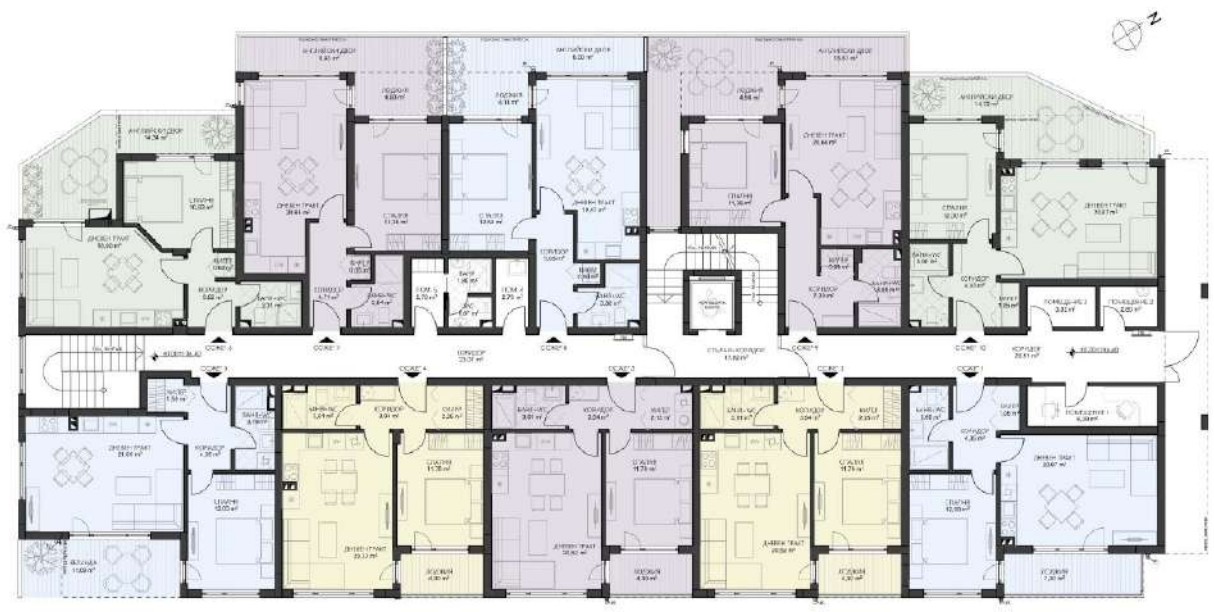
РАЗПРЕДЕЛЕНИЕ ЕТАЖ I
