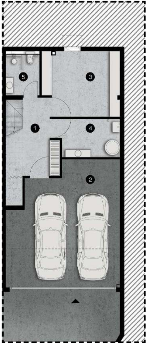
СУТЕРЕН
