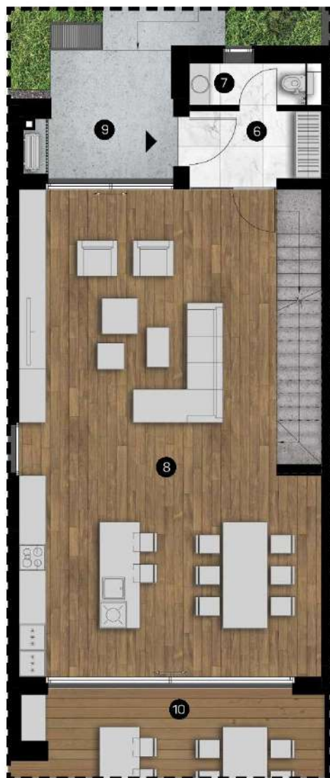
ПРИЗЕМЕН ЕТАЖ
